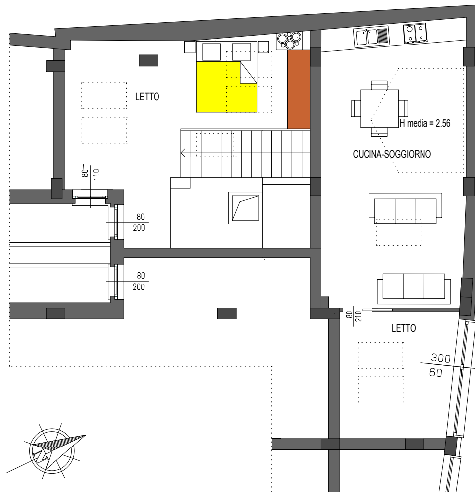
PIANTA SOTTOTETTO
