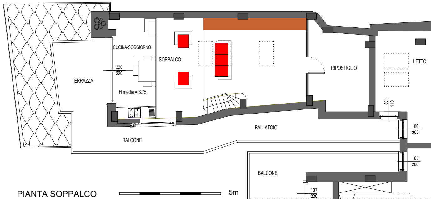
PIANTA PIANO MANSARDA TRILOCALE CON SOPPALCO (N.6)
